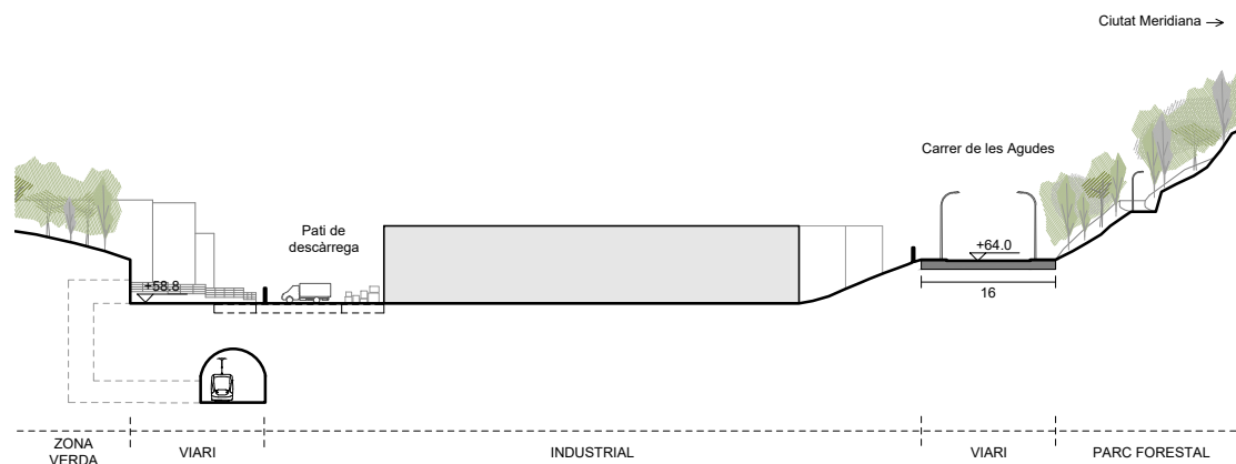
Secció CC' _ Estat actual
