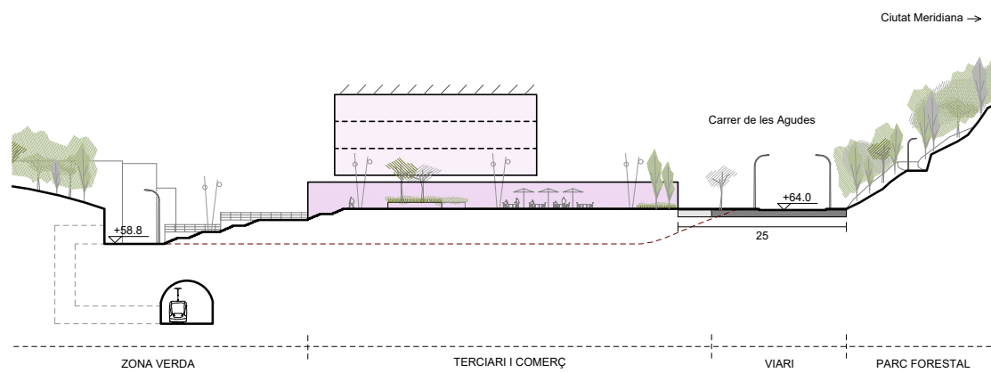
Secció CC' _ Proposta indicativa
