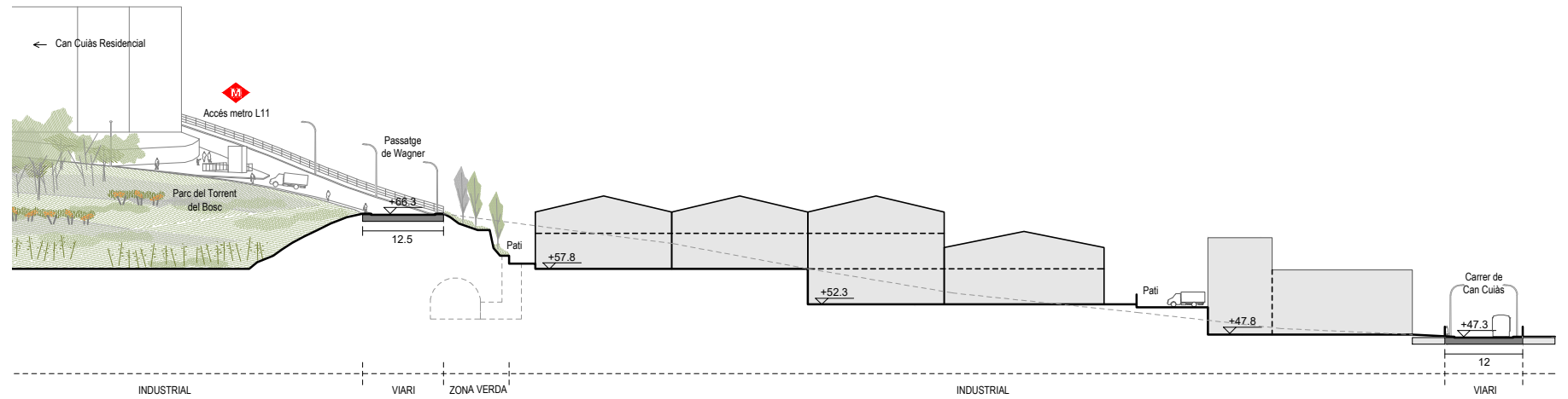
Secció DD' _ Estat actual
