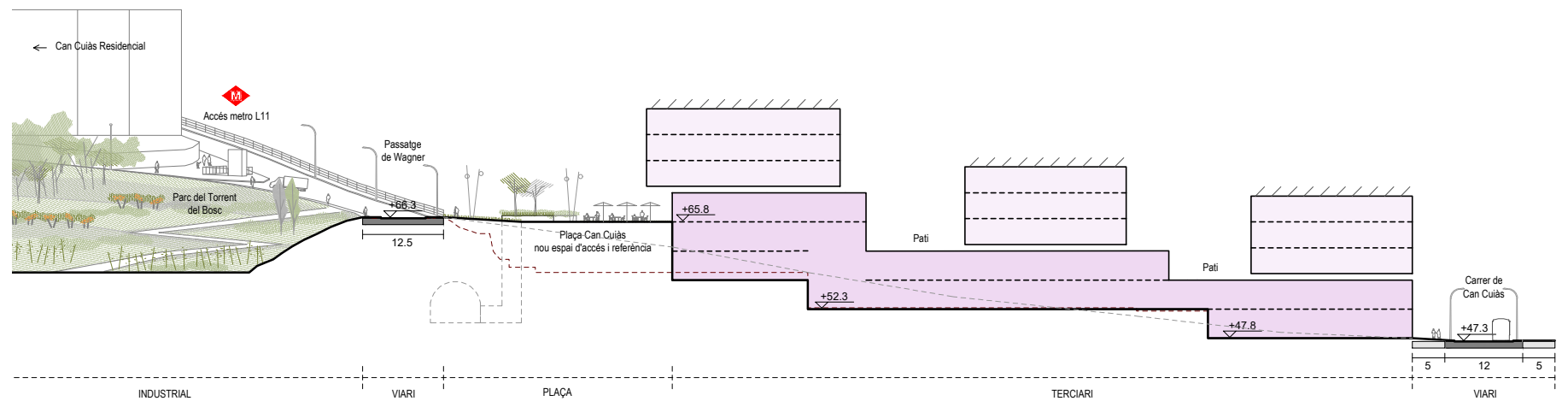
Secció DD' _ Proposta indicativa
